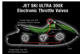
Elektronisk gasspjäll
